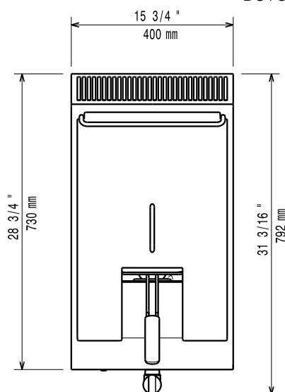
Boven aanzicht
